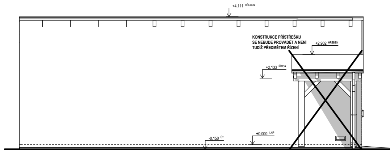
POHLED SEVEROZÁPADNÍ
