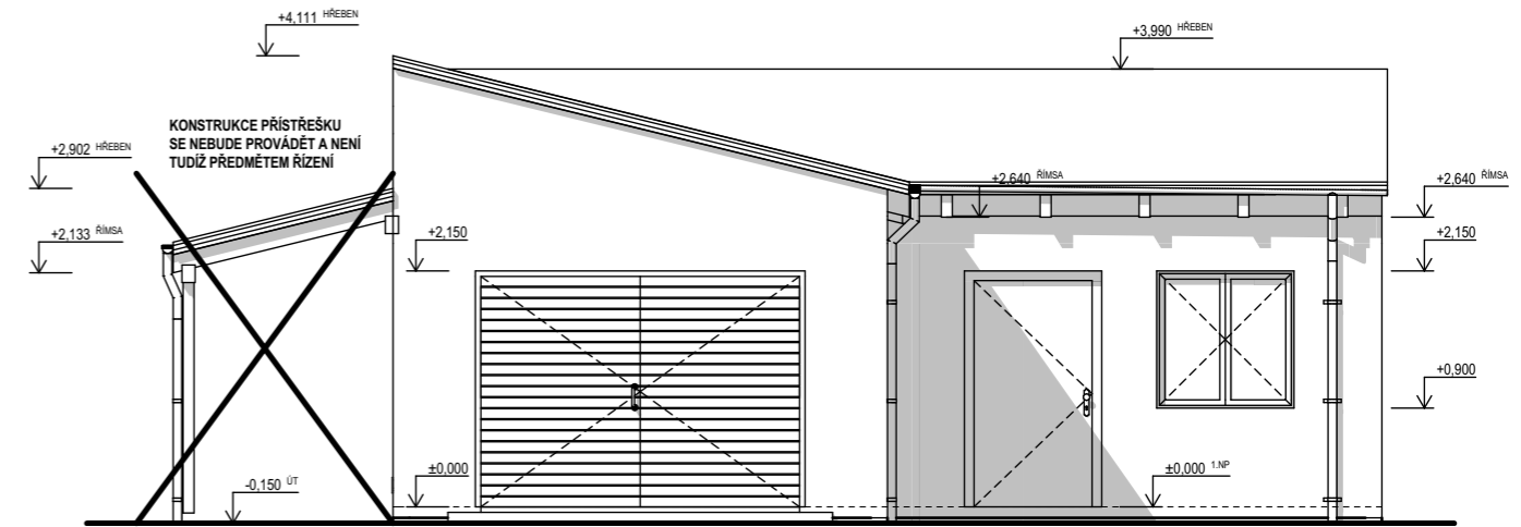
POHLED JIHOZÁPADNÍ
